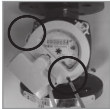
WMAP EVO 1 gancio e 1 vite
